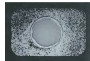
ASTROMAG (KEK)
